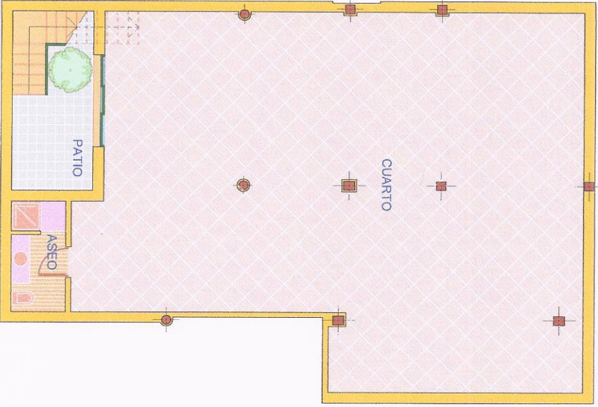
PLANTA SEMISOTANO
